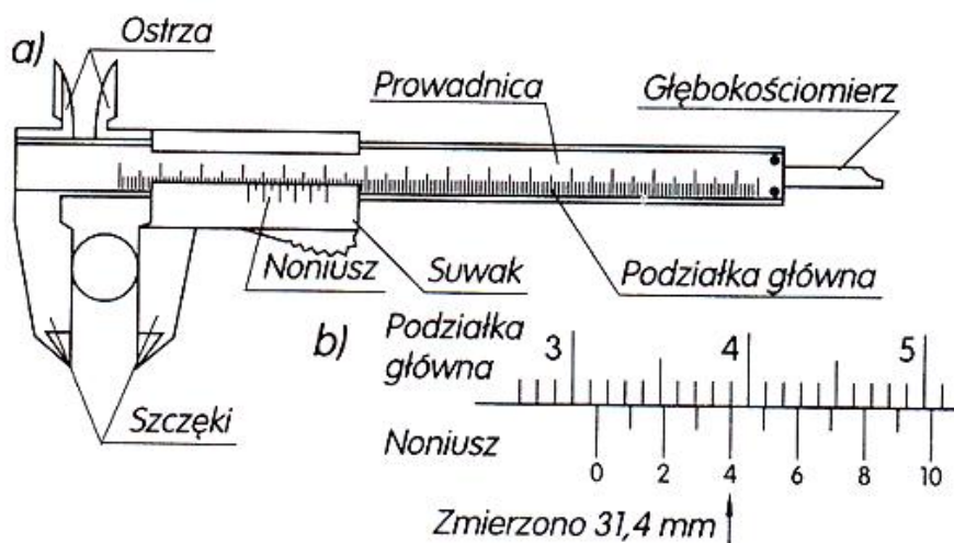
Rys. 10. Pomiar suwmiarką: a) suwmiarka, b) przykład odczytania pomiaru [6, s. 157]
