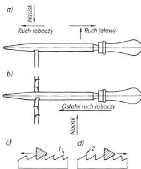
Rys. 25. Ostrzenie piły bez bocznego zaostrenia zębów: a) widok z boku, b) widok z góry, c) ostrzenie pod ząb – prawidłowe, d) ostrzenie w kierunku pochylenia zębów – nieprawidłowe [6, s. 166]
