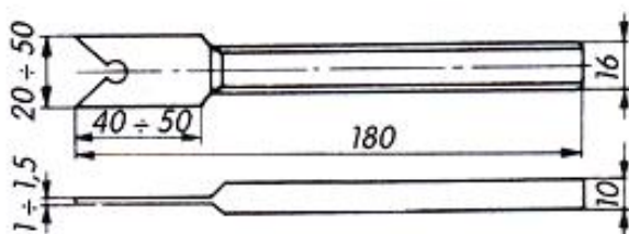
Rys. 59. Dłuto do zawiasów – szczelinowe, dwuostrzowe [6, s. 189]
