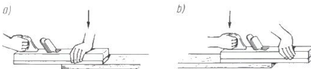
Rys. 48. Sposób ujęcia i prowadzenie spustu: a) początek posuwu, b) końcowa faza posuwu [5, s. 306]
