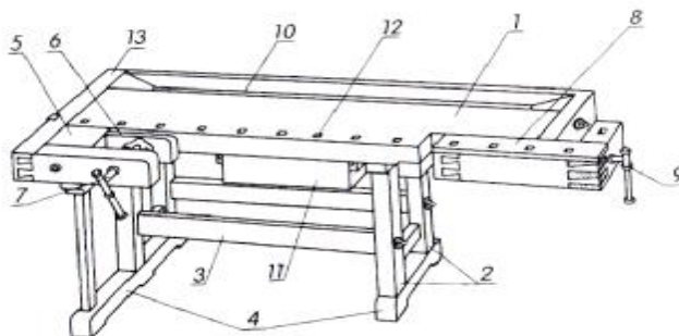
Rys. 1. Strugnica stolarska [6, s. 147]
