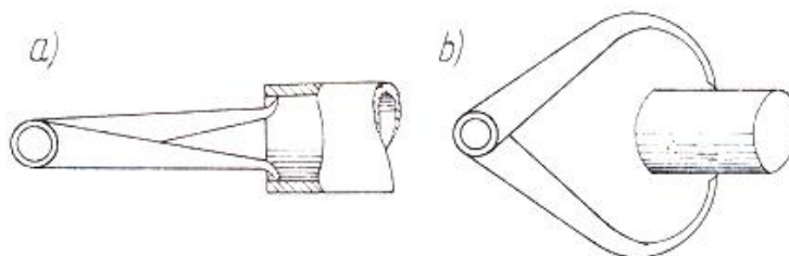
Rys.11. Macki do sprawdzania średnic: a) wewnętrzne, b) zewnętrzne [6, s. 157]
