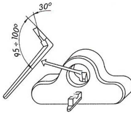
Rys. 40. Strug wyślabiak (wybiornik) [6, s. 174]
