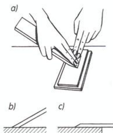
Rys. 45. Wygładzanie ostrza noża na oselce: a) sposób trzymania noża, b) i c) położenie noża przy wygładzaniu [6, s. 177]
