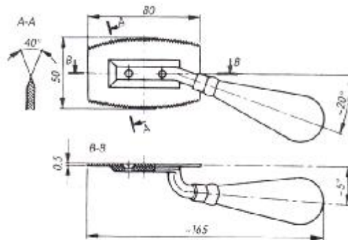
Rys. 23. Przyrznica do fornirów dwustronna [6, s. 163]
