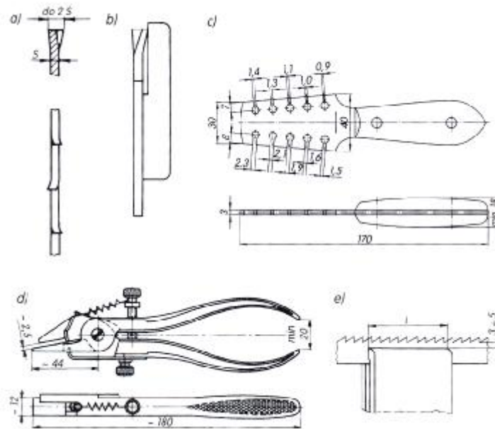
Rys. 24. Rozwieranie zębów piły: a) zęby rozwarte – przekrój poprzeczny i widok z góry, b) sprawdzian do kontroli rozwarcia zębów, c) rozwierak jednoramienny, d) rozwierak szczypcowy, e) zamocowanie brzeszczotu piły do rozwierania i ostrzenia zębów [6, s. 164]
