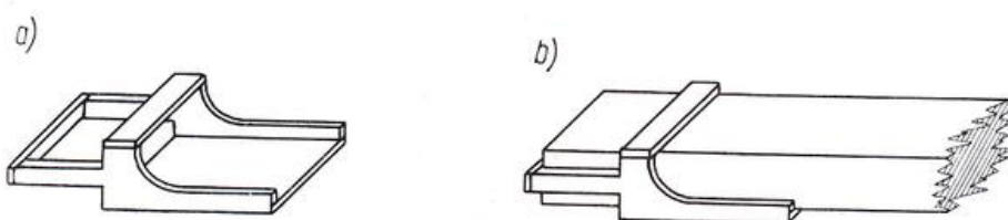
Rys. 32. Trasowanie czopów za pomocą wzornika: a) wzornik, b) element z założonym wzornikiem [5, s. 291]
