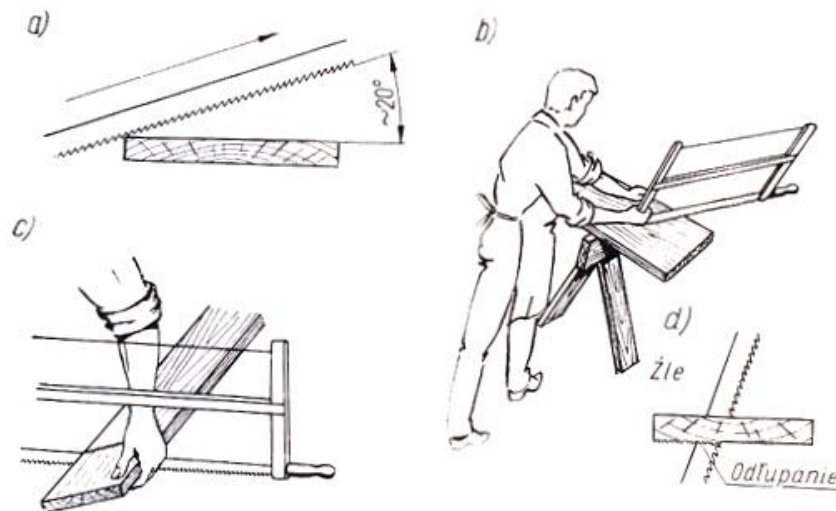
Rys. 27. Przerzynanie poprzeczną: a) faza początkowa (pierwsze pociągnięcia piłą do siebie), b) przerzynanie, c) faza końcowa, d) niewłaściwe nachylenie brzeszczotu do poziomu deski [5, s. 289]
