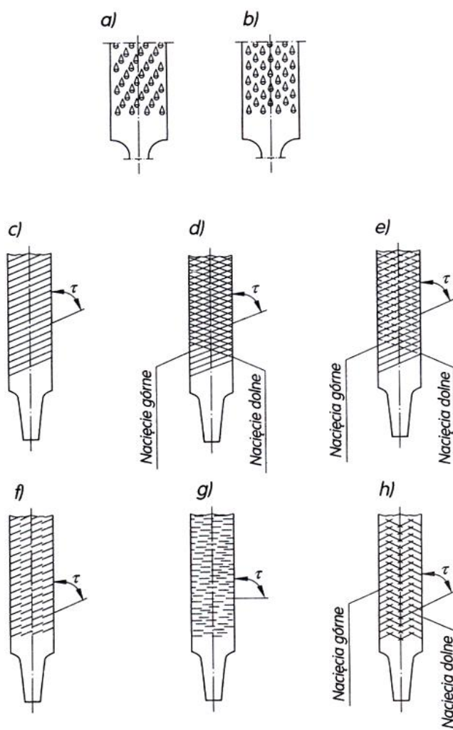
Rys. 64. Nacięcia: – tarników: a) niesymetryczne, b) symetryczne, – pilników: c) pojedyncze, d) podwójne, e) podwójne z rozdzielnymi nacięciami górnymi i dolnymi, f) i g) pojedyncze wielorzędowe, h) podwójne wielorzędowe [6, s. 192]
