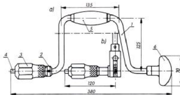
Rys. 55. Korba do świrdrów z uchwytem dwuszczkowym: a) zwykła, b) z mechanizmem zapadkowym 1 – pałak stalowy, 2 – wrzeciono, 3 – nakrętka, 4 – szczęki, 5 – uchwyt, 6 – główka [6, s. 183]
