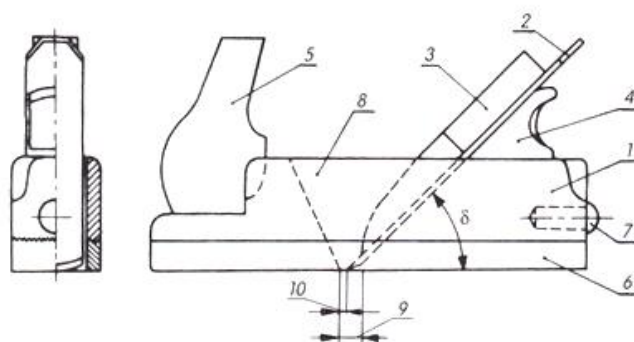
Rys. 36. Budowa struga (opis w tekście) [6, s. 170]
