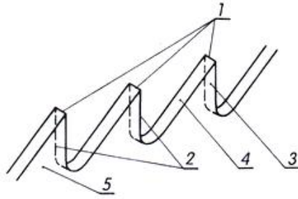
Rys. 14. Elementy zębów piły [6, s. 158]
