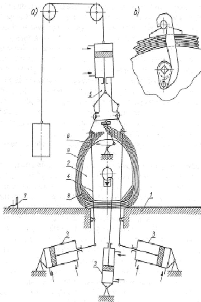
Rys. 14. Giętarko-sklejarka do ram siedziskowych krzesła, a) schemat, b) fragment formy z urządzeniem dociskowym końców pakietu: 1) stół, 2) forma, 3) siłowniki pneumatyczne, 4) ramiona, 6) mechanizm dźwigowy, 7) przekładnia, 8) wkładka, 9) taśma stalowa
