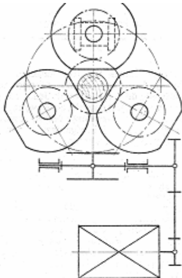
Rys. 28. Zgniatarka krążkowa do czopów walcowych Przednich nóg krzesel giętych [3, s. 273]
