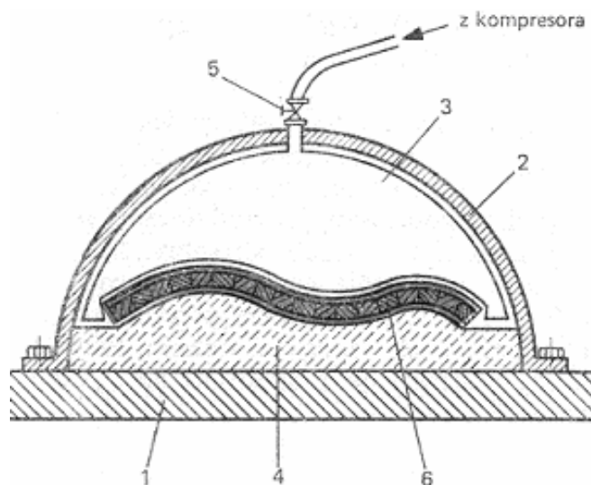
Rys. 27. Maszyna do prasowania płynnego: 1 – podstawa, 2 – obudowa metalowa, 3 – worek gumowy, 4 – forma, 5 – zawór powietrza, 6 – płyta stolarska oklejana dwustronnie fornirem [3, s. 273]
