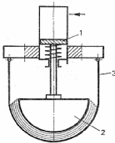
Rys. 26. Maszyna ze sztywną formą i elastycznym dociskiem za pomocą taśmy stalowej: 1 – cylinder, 2 – forma, 3 – taśma stalowa [3, s. 272]
