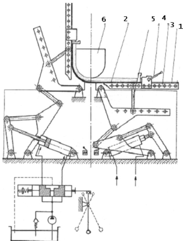
Rys. 20. Giętarka z ramionami z napędem hydraulicznym: 1 – taśma łącząca ramiona, 2 – taśma napięta na elemencie, 3 – ramię, 4 – korbowy napinacz taśmy, 5 – łącznik 6 – forma [3, s. 266]
