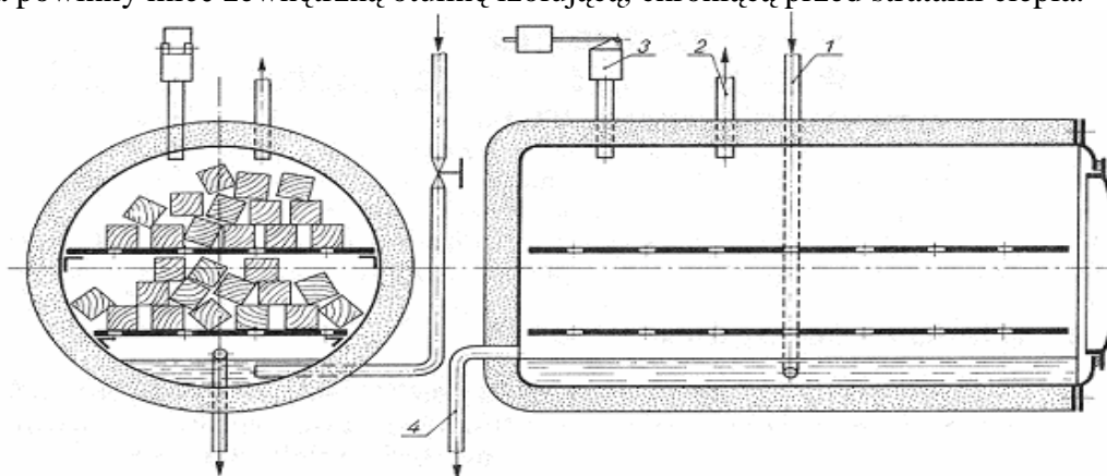
Rys. 3. Parnik do łąt giętych: 1 – przewód doprowadzający parę, 2 – przewód odprowadzający parę, 3 – zawór bezpieczeństwa, 4 – przewód odprowadzający skropliny [1, s. 253]
