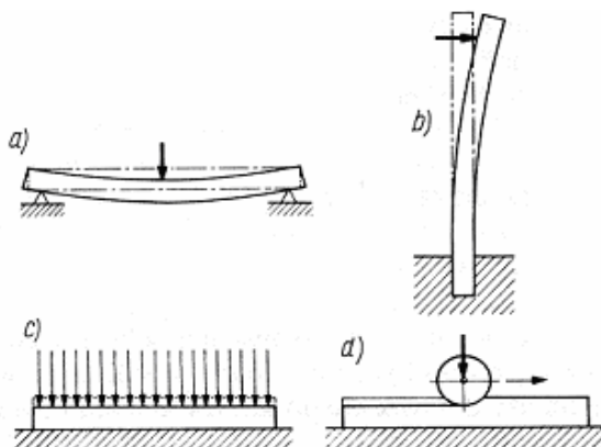
Rys. 1. Przyłożenie sił do elementu przy: a), b) zginaniu, c), d) zginiataniu [1, s. 254]
