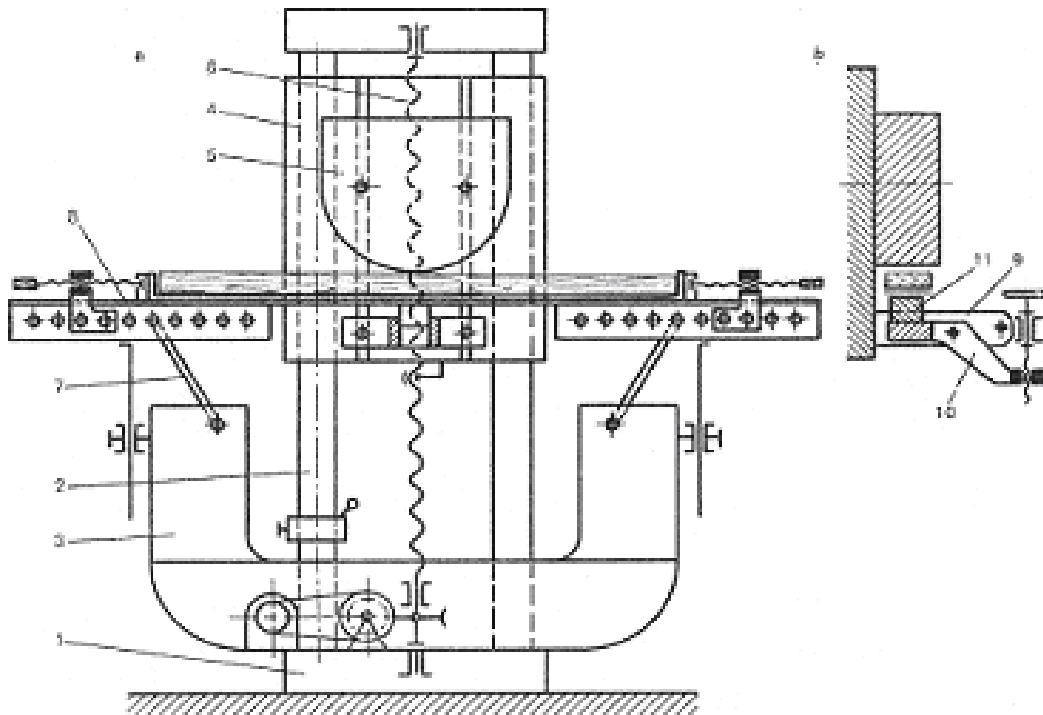
Rys. 21. Giętarka z ramionami z przesuwaną formą: a – widok z przodu, b – zespół dociskający element do form; 1 – podstawa, 2 – słupy, 3 – wspornik kadłuba, 4 – suport, 5 – forma, 6 – śruba pociągowa, 7 – łączniki, 8 – taśma, 9 – wspornik, 10 – dźwignia 11 – kostka naciskowa [3, s. 268]
