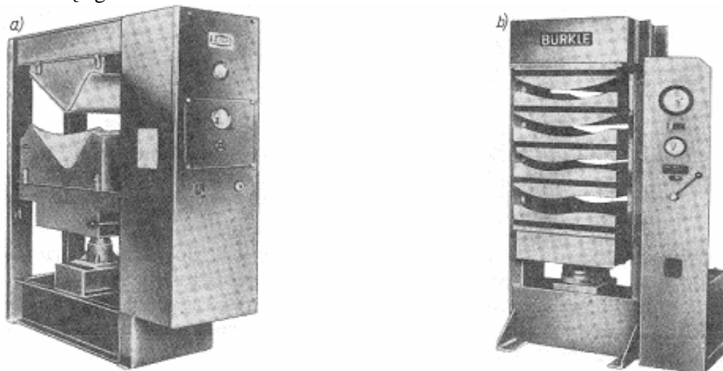
Rys. 12. Giętarko-sklejarki: a) do pojedynczych elementów o głębokich krzywiznach, b) do kilku elementów o niewielkich krzywiznach [2, s. 269]
